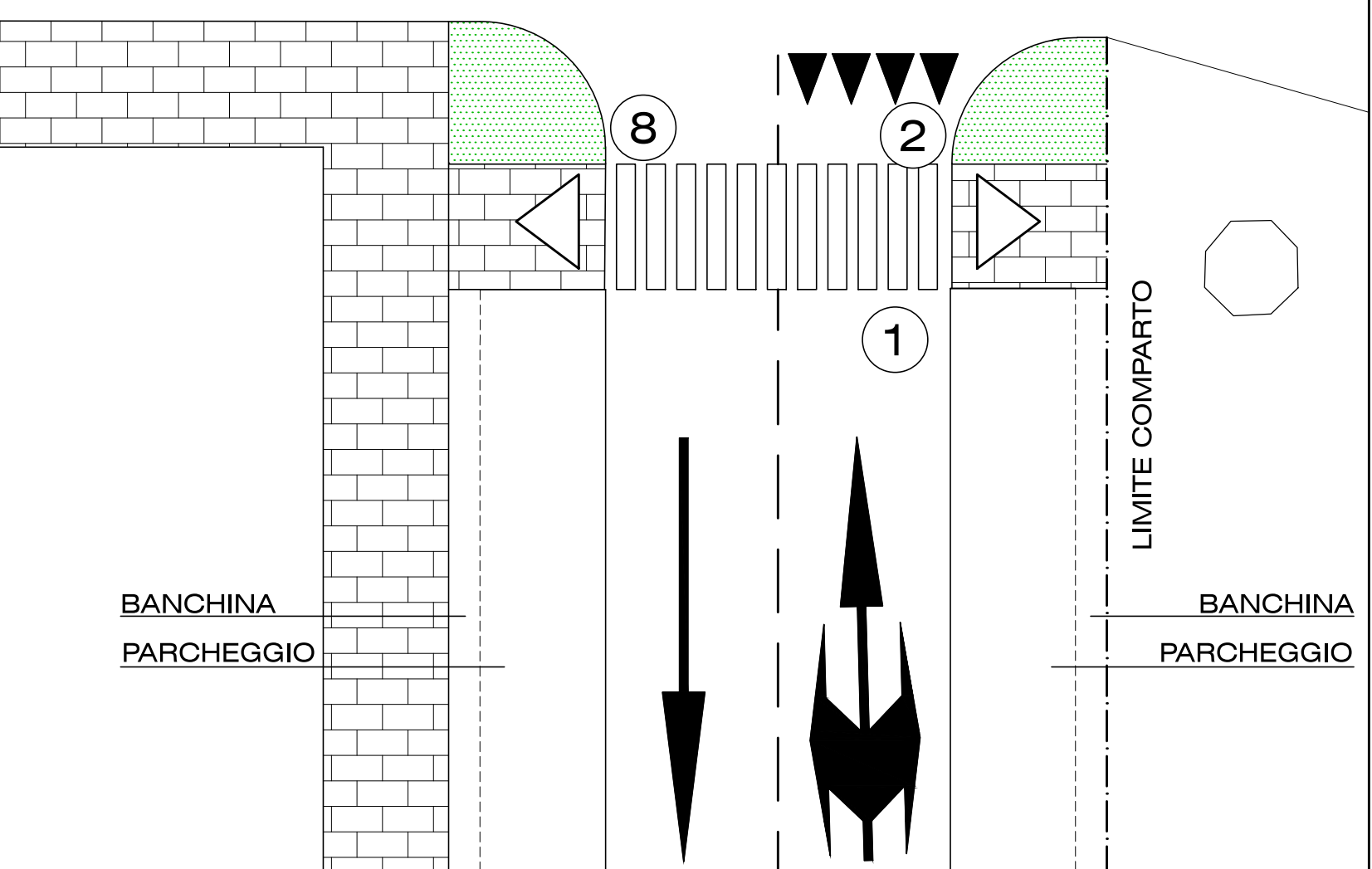
PARTICOLARE 2 SCALA 1:100
