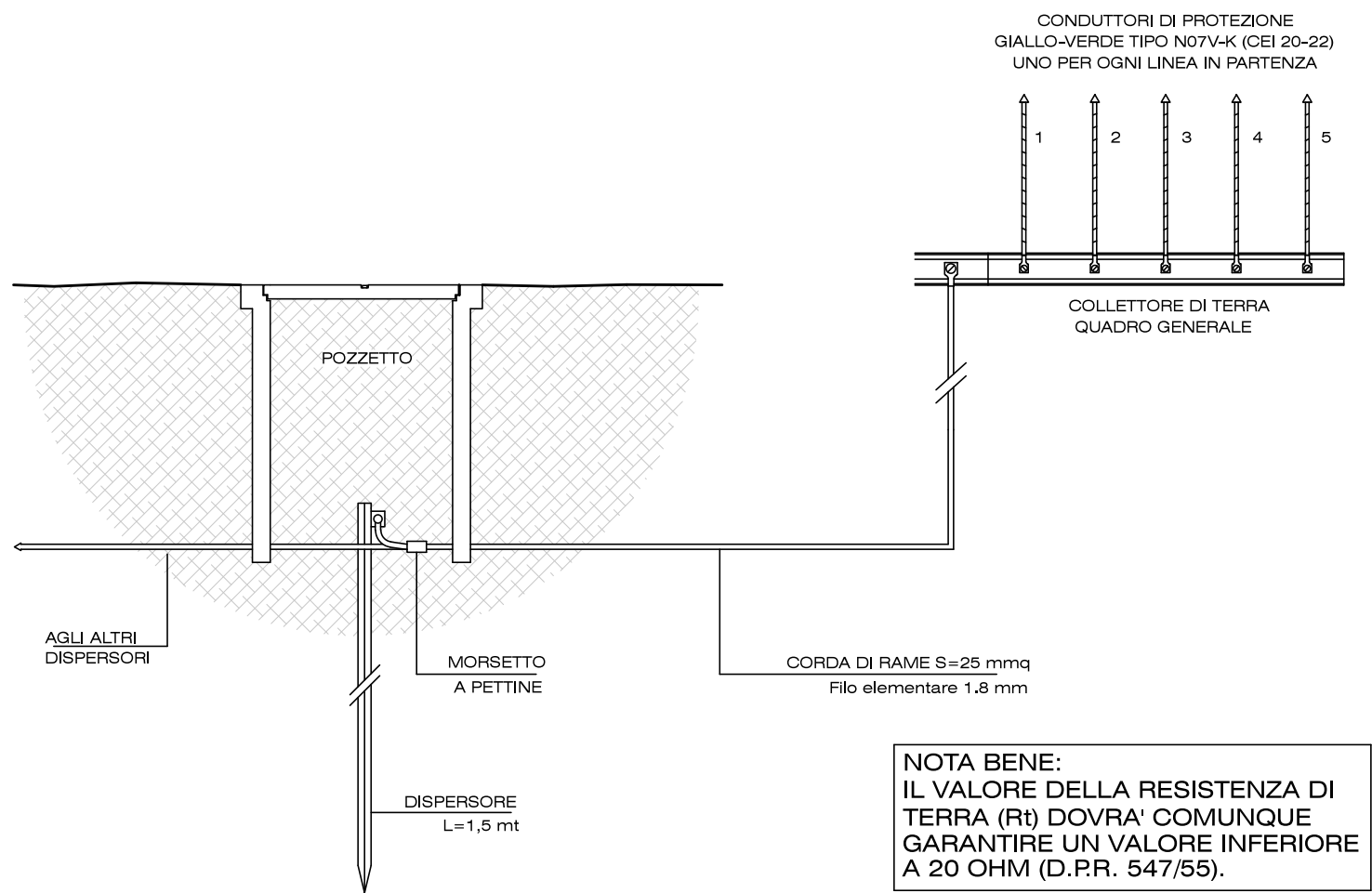
IMPIANTO DI TERRA - 1:20
